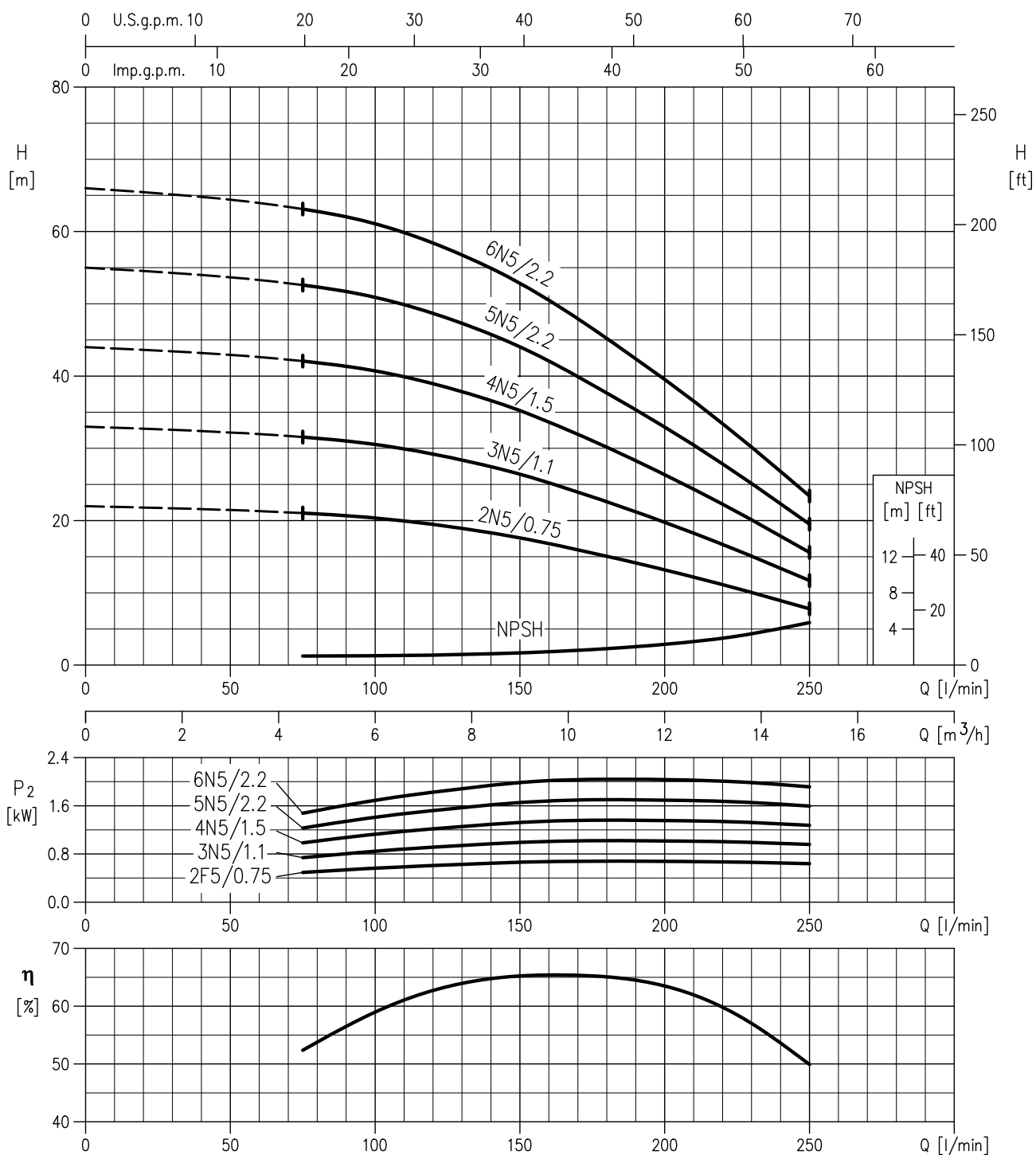
EVM(.)10 MEI > 0.70 - Impeller diameter =96 mm
